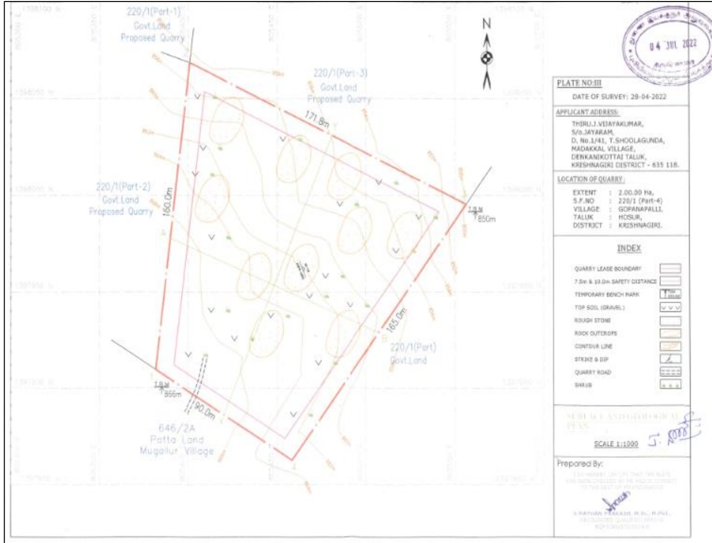
படம் 2.2 சுரங்க குத்தகை திட்டம்
