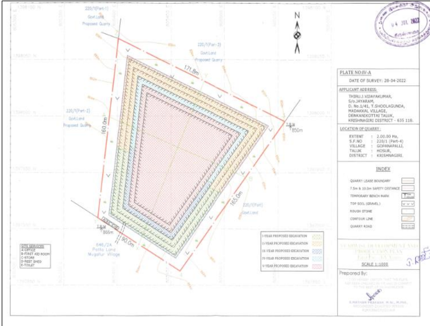
படம் 2.3 ஆண்டு வாரியான உற்பத்தி மேம்பாடுத் திட்டம்
